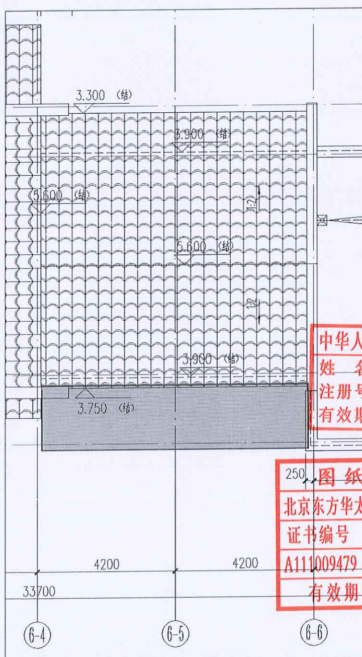
原 6#楼屋顶平面
