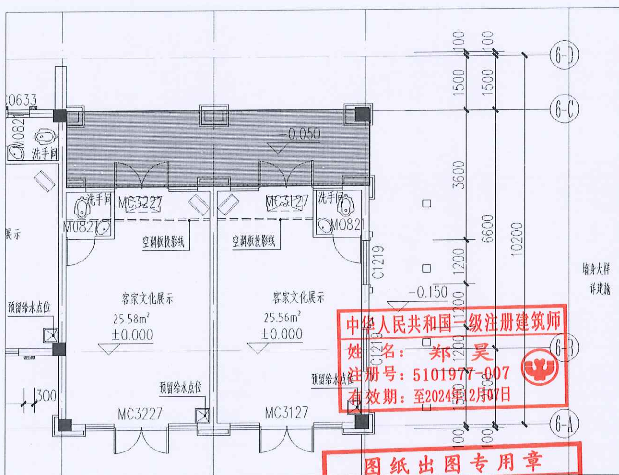
原 6#楼一层平面
