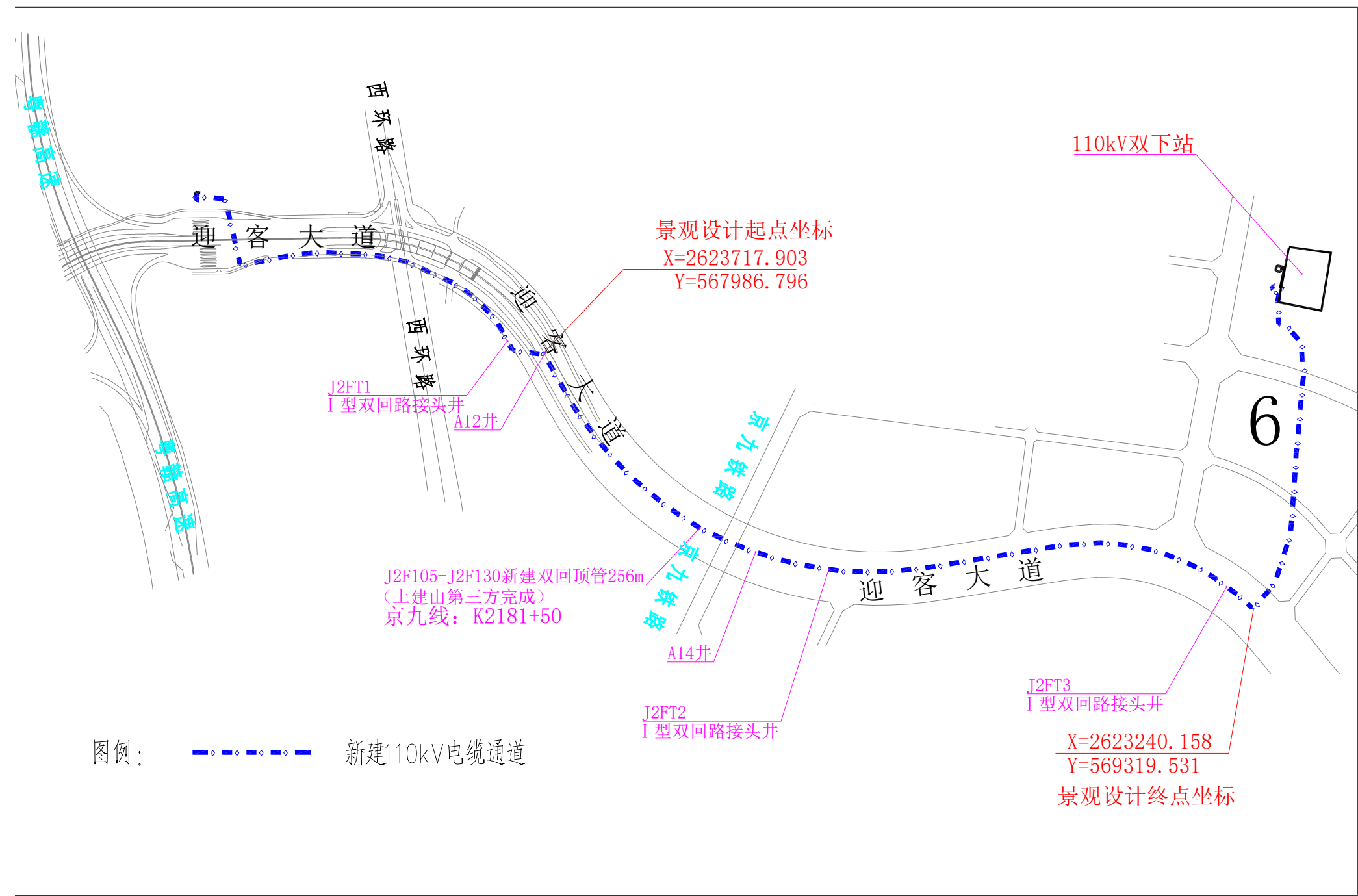
附件 1: 河源 220 千伏万绿湖输变电工程桂山迎客大道段新建电缆通道线路路径图
